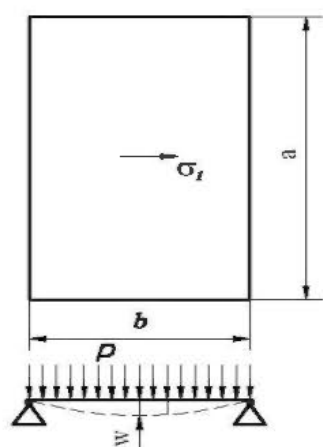
а) свободно опертая пластина
