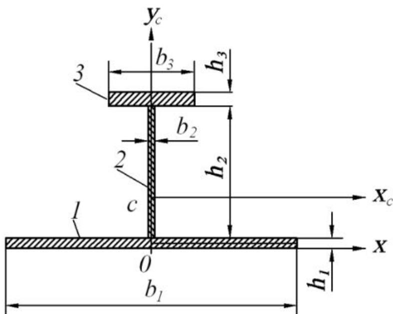
1 – присоединенный пояс; 2 – стенка тавровой балки; 3 – полка тавровой балки
